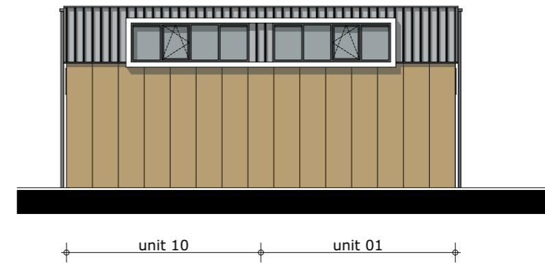
OOSTGEVEL
