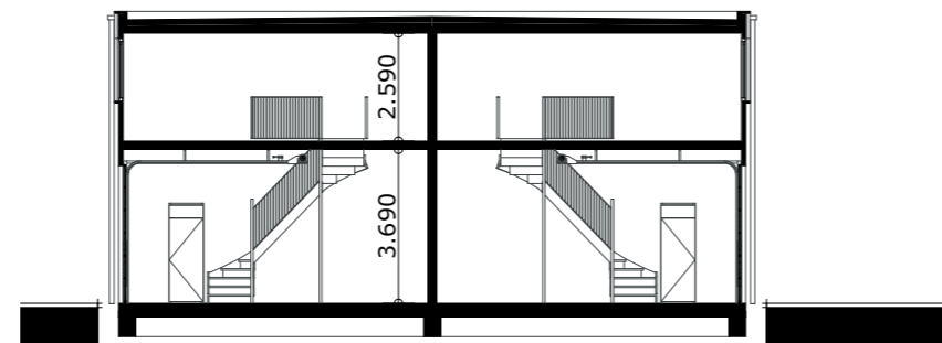
DOORSNEDE B-B
