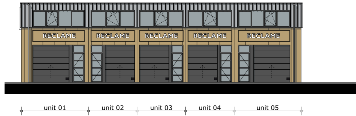
NOORDGEVEL
