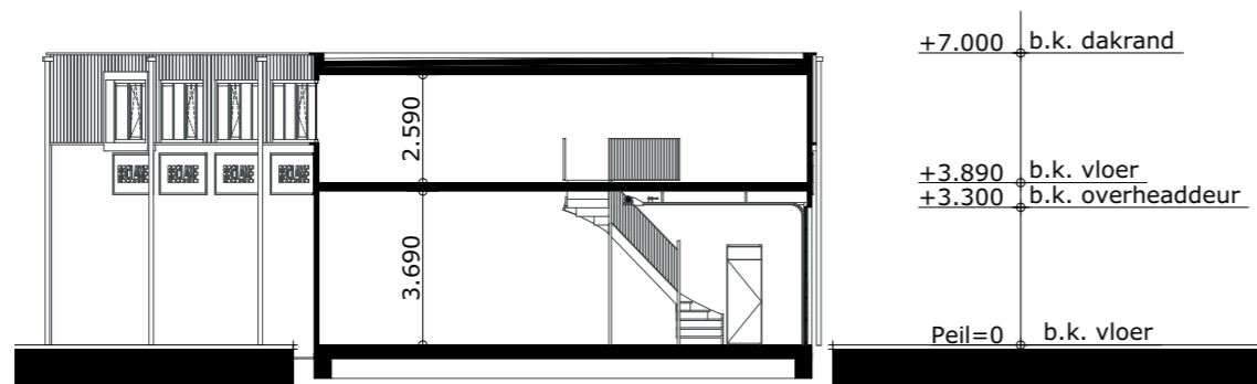
DOORSNEDE B-B
