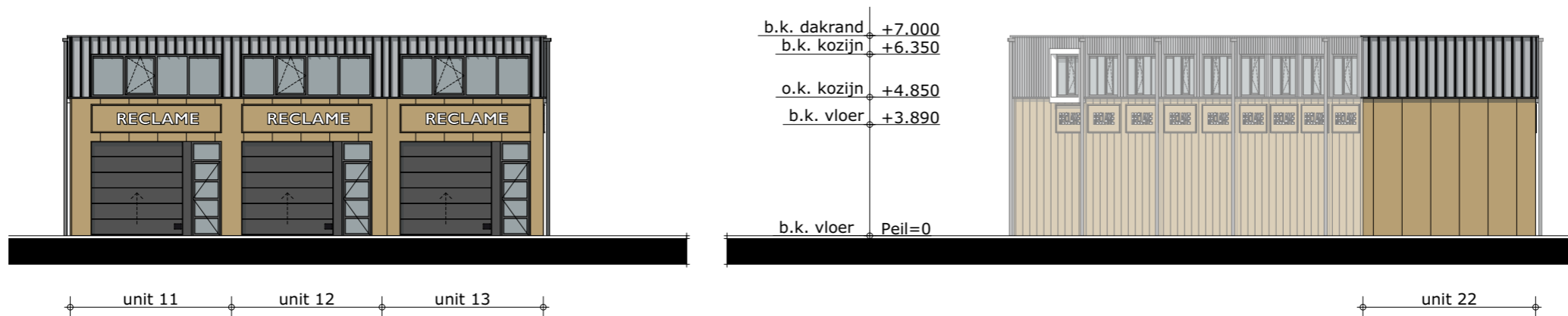
NOORDGEVEL
