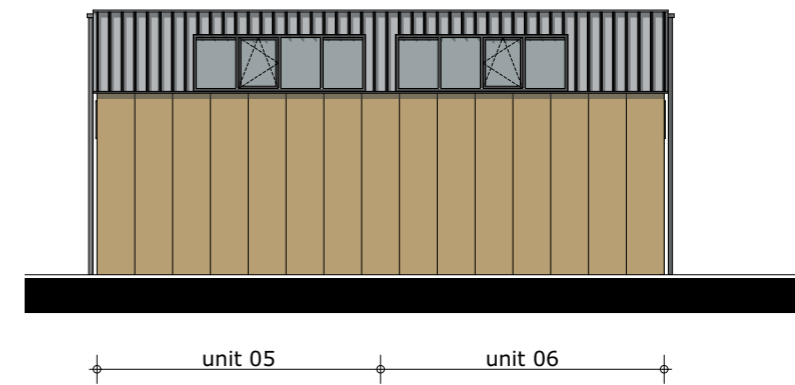
WESTGEVEL
