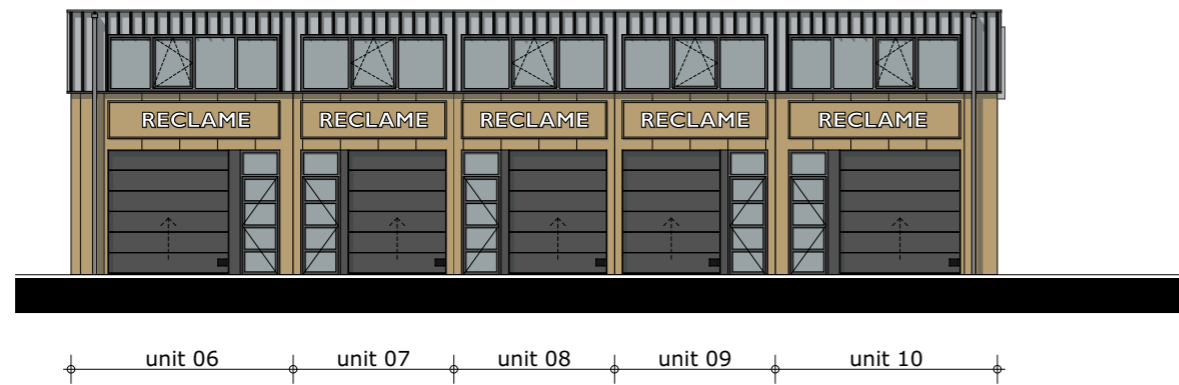
ZUIDGEVEL
